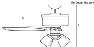
Fan Dimensions in Inches
